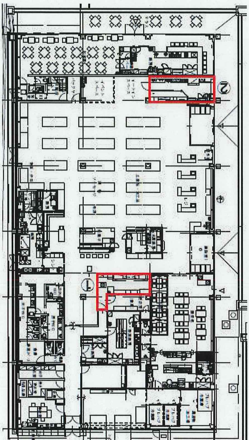
道の駅日光「日光街道ニココ本陣」商業施設テナント 物件1、物件2 平面図
